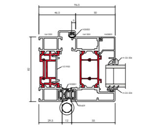
F82 Jamb
