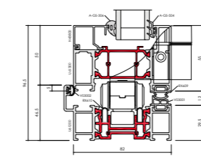
F82 Cill
